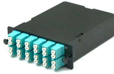
24芯LC MPO-24LC多模转接盒
